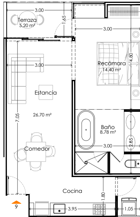
Planta 1er Nivel
